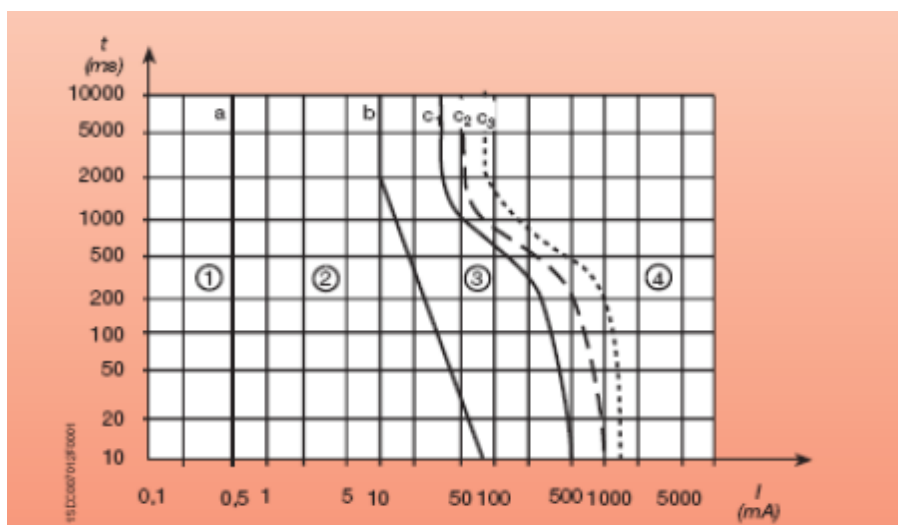
Figura 5.2 – Zone di pericolosità della corrente elettrica alternata (15-100Hz)
