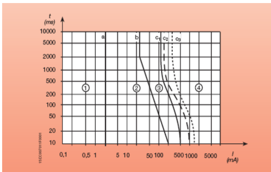
Figura 5.1 - Zone di pericolosità della corrente continua
